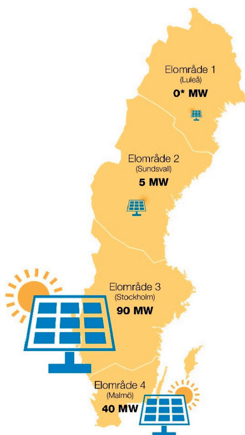
Figur 3. Installerad effekt över nätanslutna solcellsanläggningar per elområde 2016, MW. Totala effekten i figuren ovan är lägre än Sveriges totala effekt då ett visst bortfall sker på grund av sekretess. *Elområde 1 har en installerad effekt om ungefär 100 kW.
